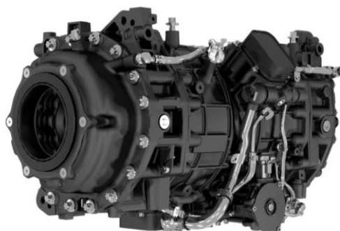
菲亚特动力科技 (FPT Industrial) eAX 600-R 后电驱动桥
